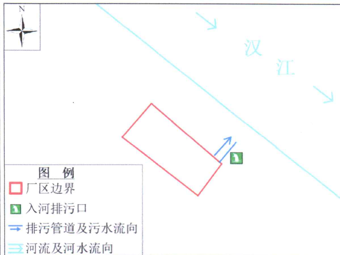
污水排放路径图（排污单位-排污管线-入河排污口-受纳水体）：
